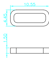
防水圈图示
